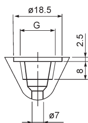
Вид "А"
