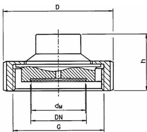
Конструкция с накидной гайкой
