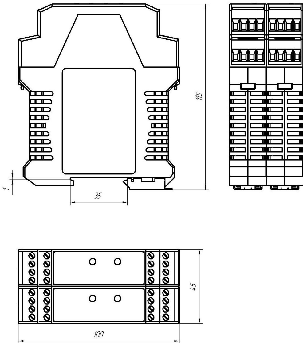
Рисунок Б.2 – Габаритные размеры Источника ЭЛМЕТРО-ИПТ-4
