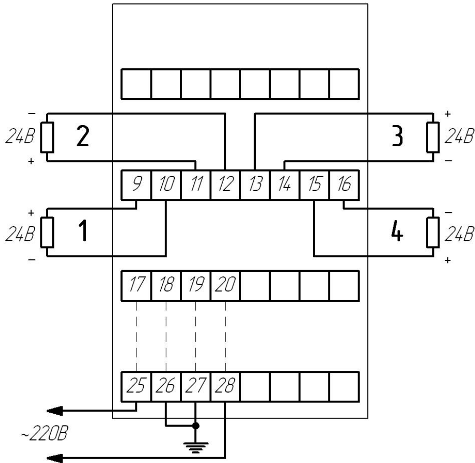
Рисунок В.2 – Схема подключения ЭЛМЕТРО-ИПТ-4
