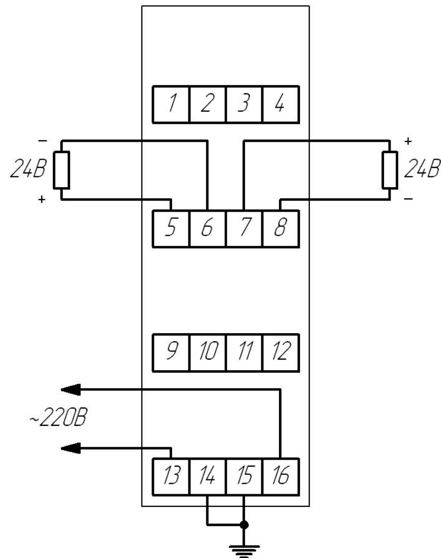
Рисунок В.1 – Схема подключения ЭЛМЕТРО-ИПТ-2
