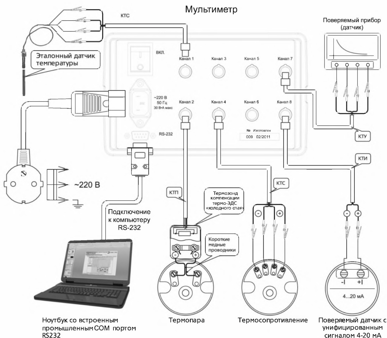
Рис. 1. Схема подключения мультиметра к различным СИТ
