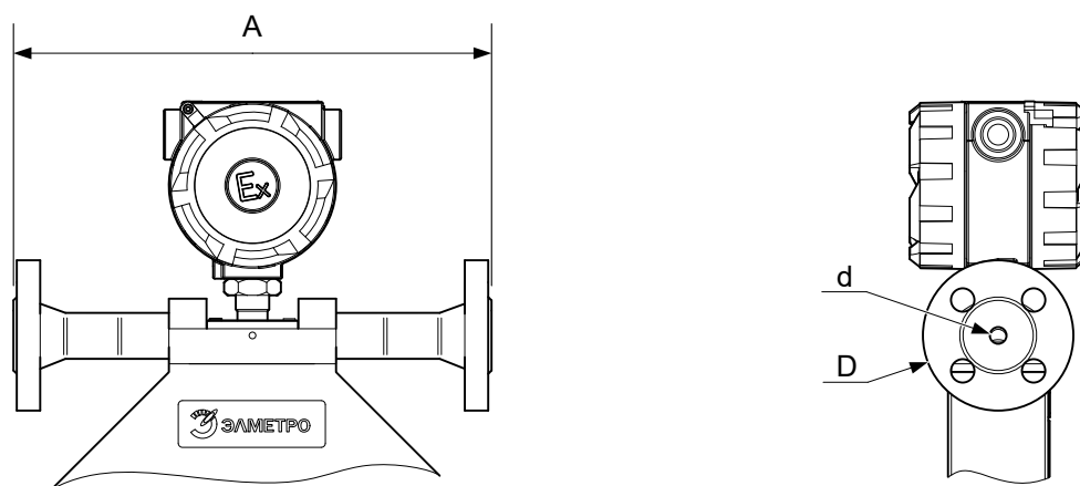
Рисунок Б.5 – Габаритные размеры датчика S010, S015 с фланцевым присоединением
