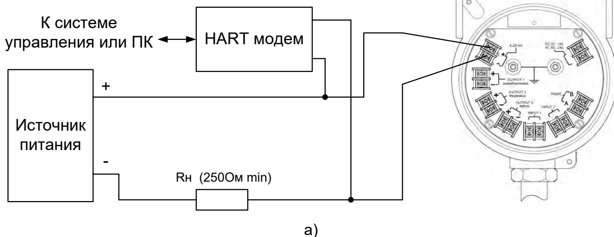
Расходомер Элметро-Фломак
