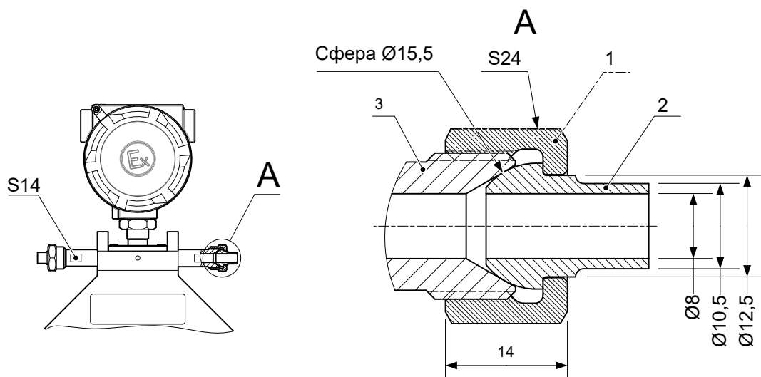
Рисунок 2.4 – Монтаж датчика со штуцерным присоединением (датчики S002, S003, S005, S010, S015), размеры указаны для S005
