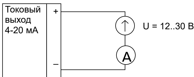
Рисунок 2.23 - Подключение измерителя тока к токовому выходу
