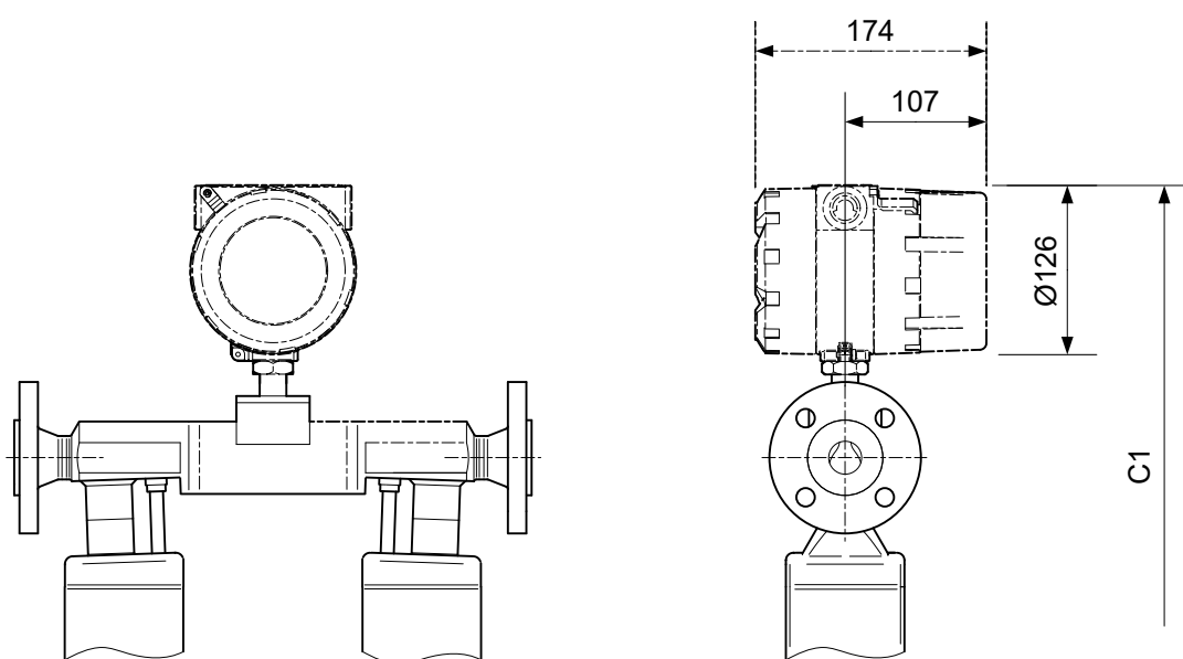
Рисунок Б.6 – Габаритные размеры датчиков, исполнение по компоновке М
