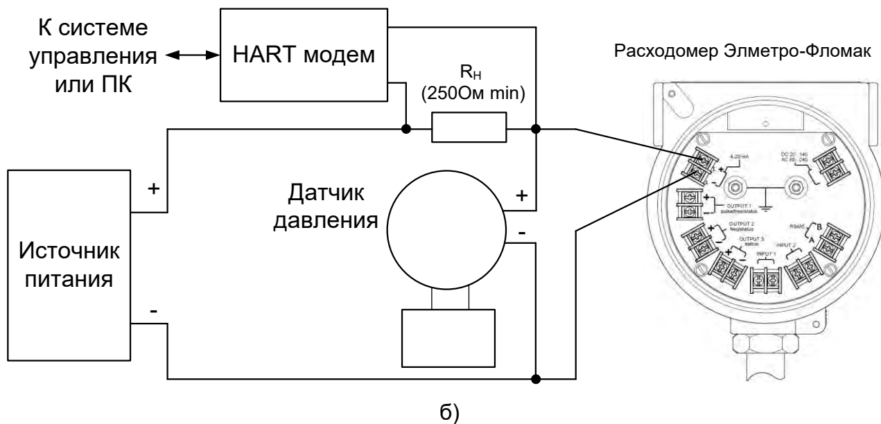
Рисунок В.4 – Подключение датчика давления для компенсации влияния избыточного давления среды на измерение массового расхода и плотности: а) датчик давления работает в монопульсном (Burst) режиме; б) датчик давления отвечает на запросы Мастер-устройства (АСУ, коммуникатора или ПК с HART-модемом)
