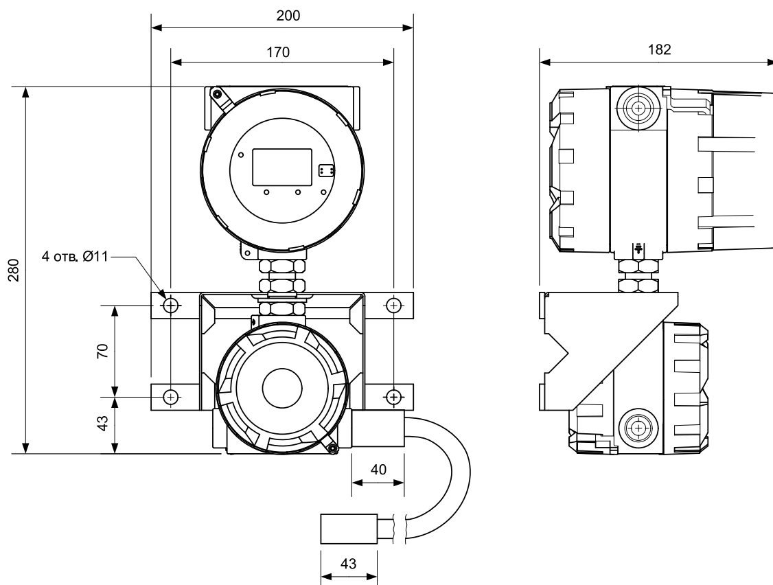
Рисунок Б.6 – Электронный преобразователь (исполнение по компоновке S), модуль процессора (исполнения по компоновке R, RS) на кронштейне
