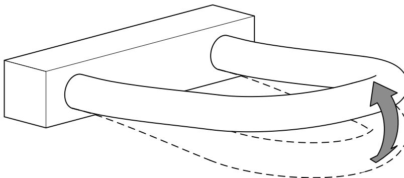
Рисунок - 1.7 – Колебания трубы датчика
