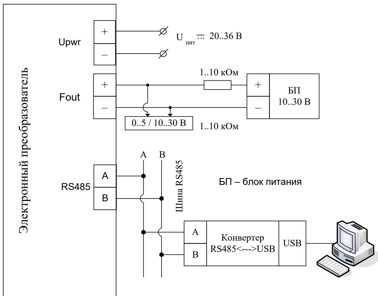
Рисунок В.2 – Схема подключения расходомера к внешним устройствам
