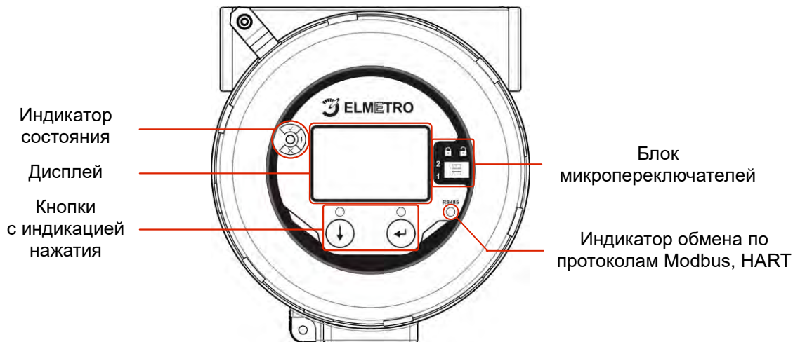
Рисунок 2.13а - Лицевая панель модуля процессора в исполнениях по компоновке I, R, S, RS, M
