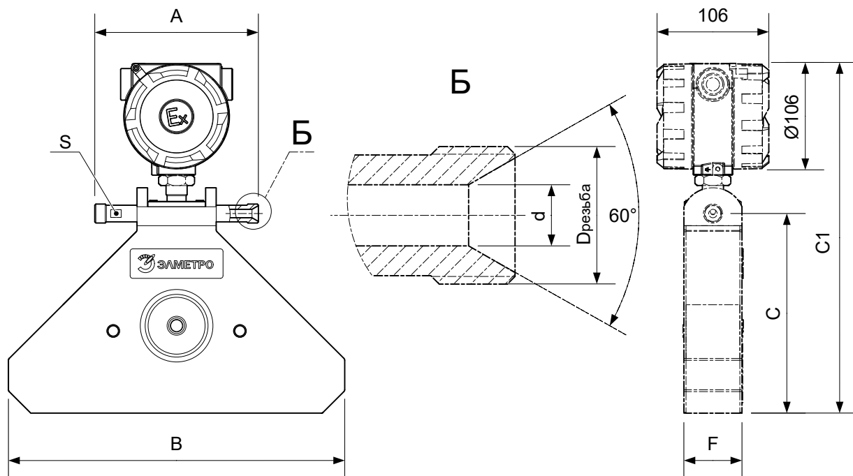
Рисунок Б.4 – Габаритные размеры датчиков S002, S003, S005, S010, S015 со штуцерным присоединением
