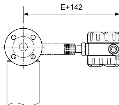
Рисунок Б.3 – Габаритные размеры датчиков, температурное исполнение S, T
