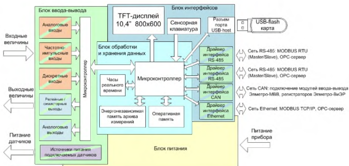
Рис. 1. Структурная схема регистратора
