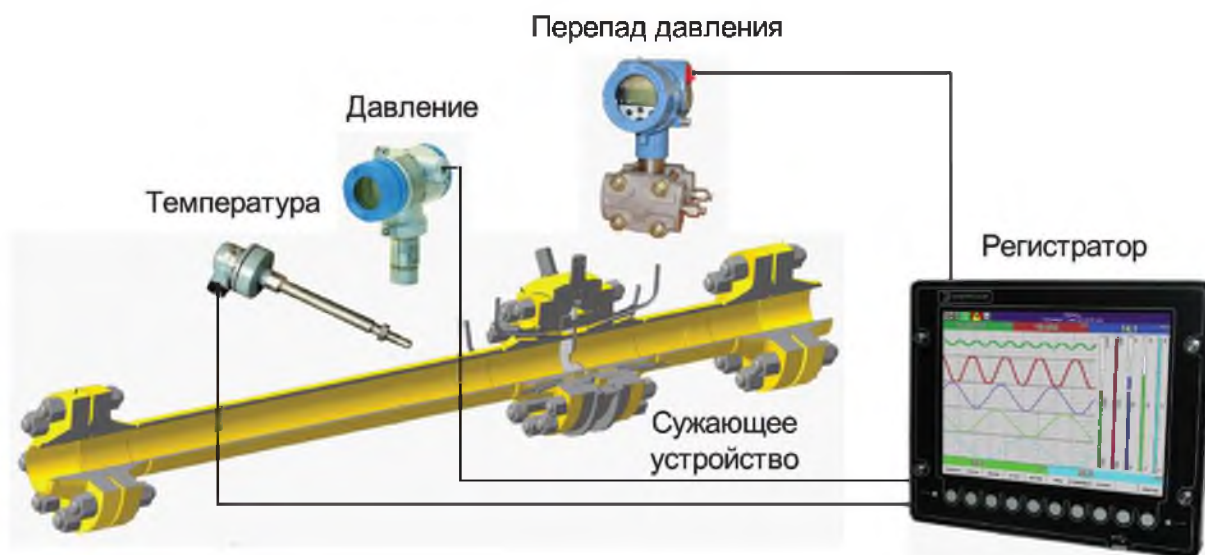
Пример 2. Измерение расхода по методу перепада давления
