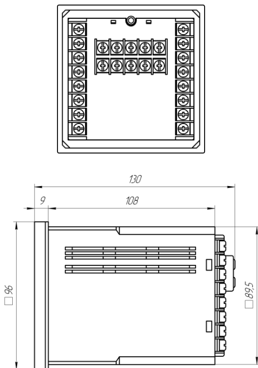
Рисунок А.1 — Общий вид и габаритные размеры.
