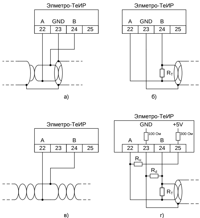
Рисунок В.2 – Варианты включения регулятора Элметро-ТеИР в сеть RS-485: а) включение при использовании экранированной витой пары; б) включение оконечного устройства с терминатором R_T (120 Ом в соответствии со стандартом RS-485); в) включение при использовании неэкранированной витой пары; г) включение оконечного устройства с терминатором R_T и смещающими резисторами R_u , R_d (смещающие резисторы определяют состояние линии, если ни один из передатчиков в сети не активен).
